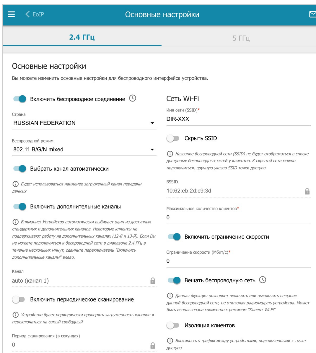
Рисунок 121. Основные настройки беспроводной локальной сети в диапазоне 2,4 ГГц.
