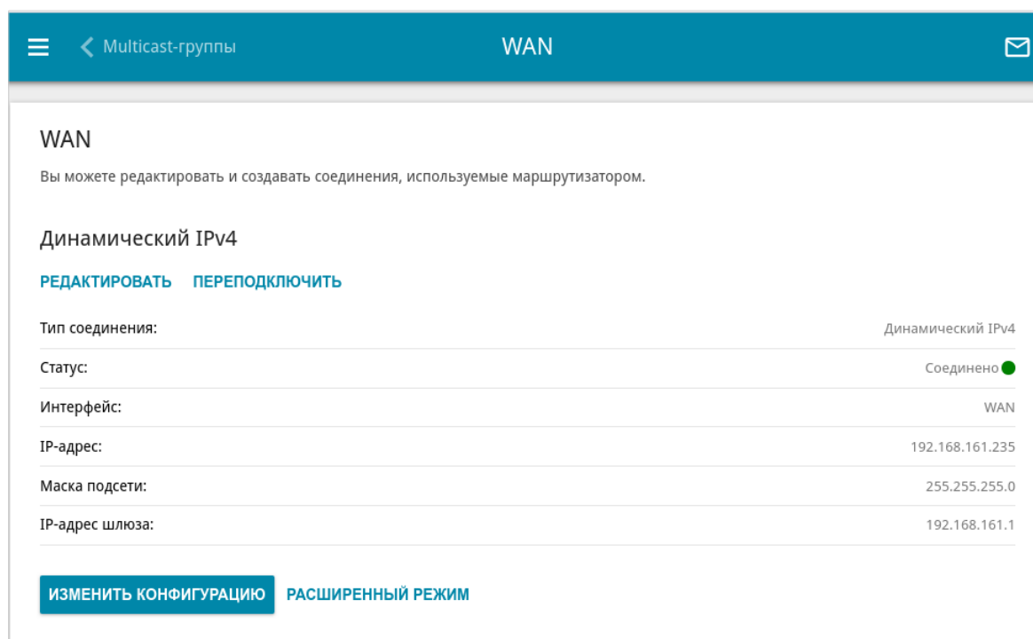
Рисунок 67. Страница Настройка соединений / WAN . Упрощенный режим.
