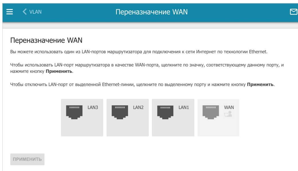
Рисунок 137. Страница Дополнительно / Переназначение WAN .
