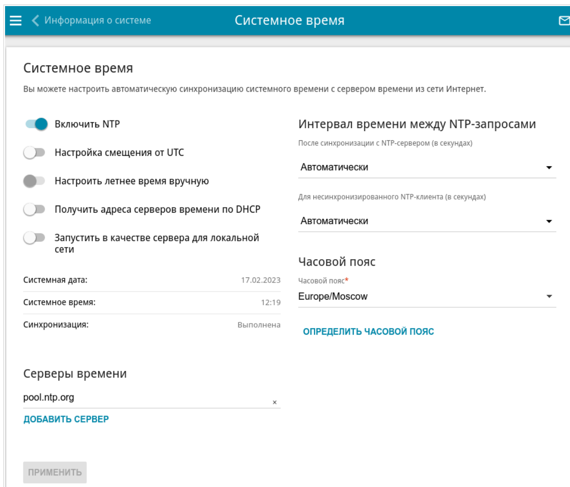
Рисунок 184. Страница Система / Системное время .
